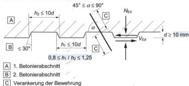
Bild 6.8 – Beispiele für Fugen
